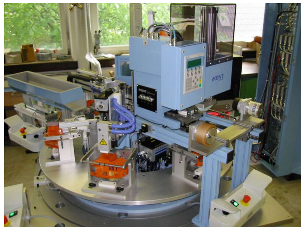
Gesamtanlage zur Bedruckung von Kunststoffteilen, mit integrierter Corona-Vorbehandlungsstation.
