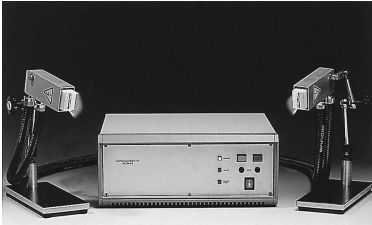
Corona mit Doppelkopf (Stative sind nicht im Lieferumfang enthalten)
