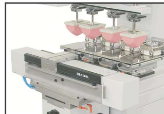
2-4 Farben Verschiebetisch
