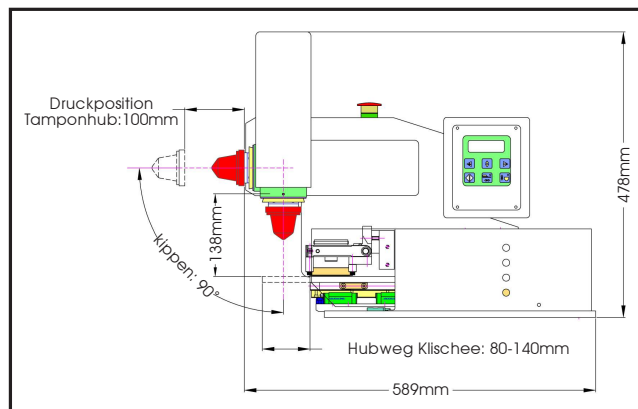
Alien 100R - Kippkopfmachine
