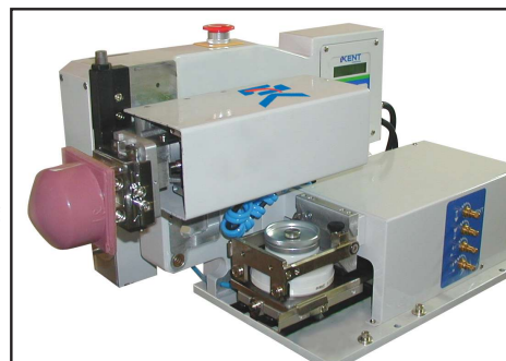
Alien 100R - Kippkopfmachine
